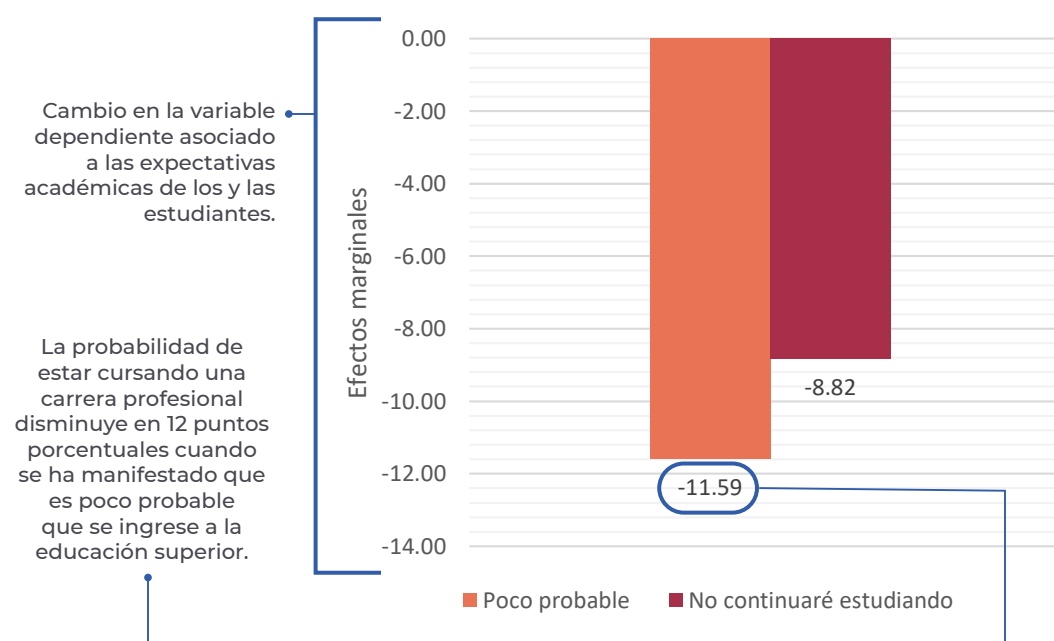
Figura 5. Ejemplo de la estimación de los efectos marginales de un modelo de regresión logística de probabilidad
