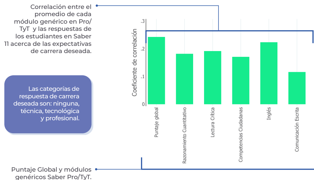
Figura 4. Ejemplo del análisis para las correlaciones policóricas
